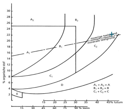
Afbeelding VII.2 Textuur/organische stoffeisen in afhankelijkheid van gebruiksdoeleinde (CROW-RAW 2015 besteknorm 51.06.01
