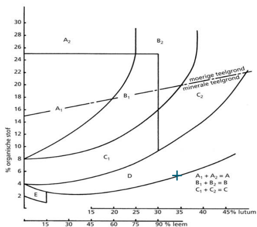
Afbeelding VII.1 Textuur/organische stofeisen in afhankelijkheid van gebruiksdoeleinde (CROW-RAW 2015 besteknorm 51.06.01 Teelgrond, 05)
